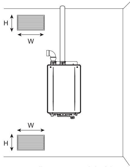
Ouvertures alimentant en air intérieur.
